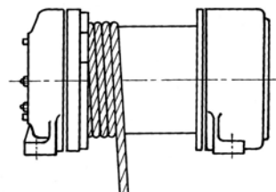
余巻き3巻以上確保のこと
