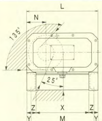
右側面図 封鎖又はロープ解は可能範囲
