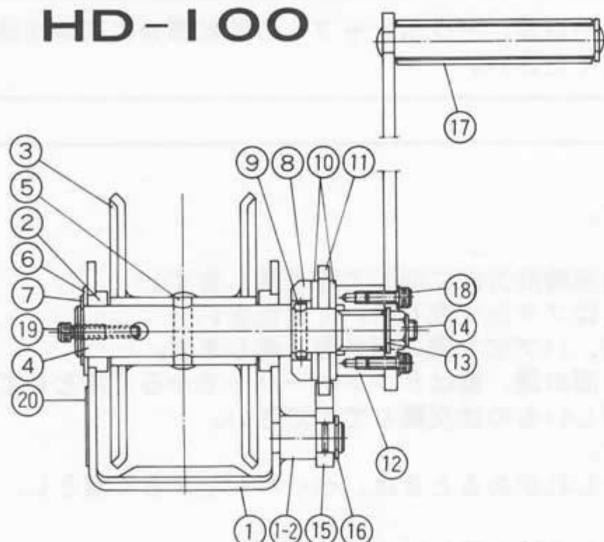
HD-100 部品表
